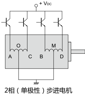
2相（单极性）步进电机
