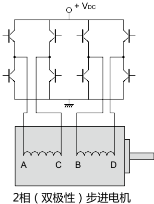
2相（双极性）步进电机
